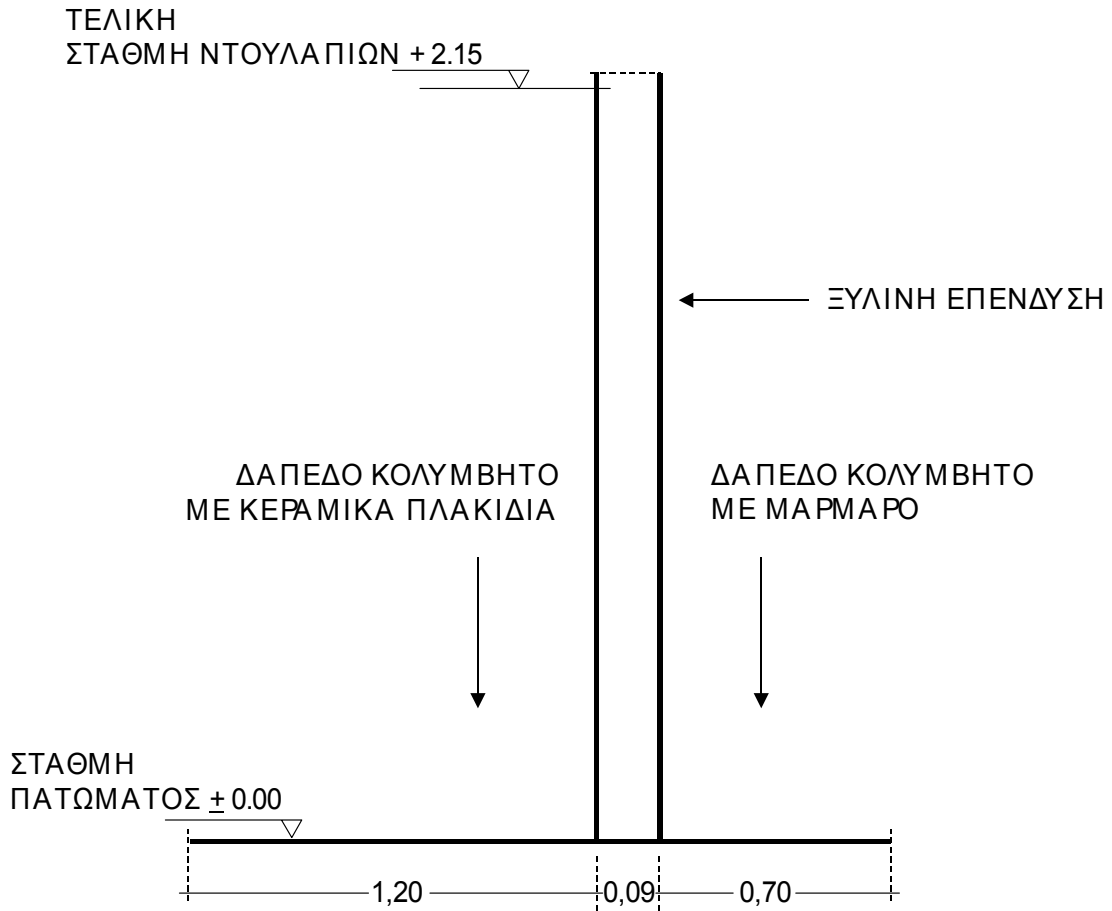
ΣΚΑΡΙΦΗΜΑ ΤΟΜΗΣ (δεν είναι υπό κλίμακα)
